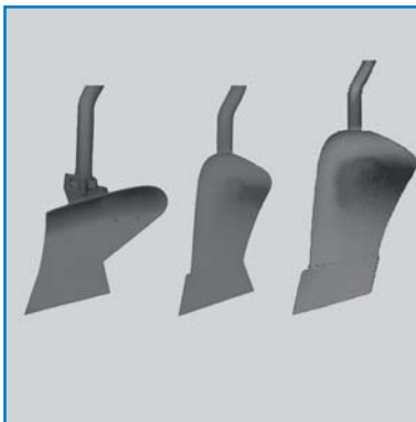
Vorschäler mit Vari-Fix oder Rundstiel
